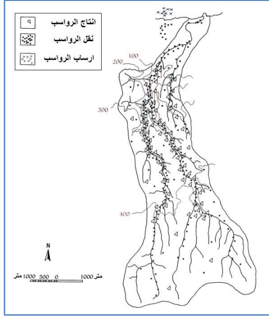
شكل (10) الآليات المقترحة لإنتاج ونقل وارساب الرواسب في وادي الرجل بعد عملية ارساب رواسب المصاطب..
