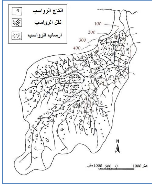
شكل (7) الآليات المقترحة لإنتاج ونقل وارساب الرواسب في وادي مرقص بعد عملية ارساب رواسب المصاطب.
