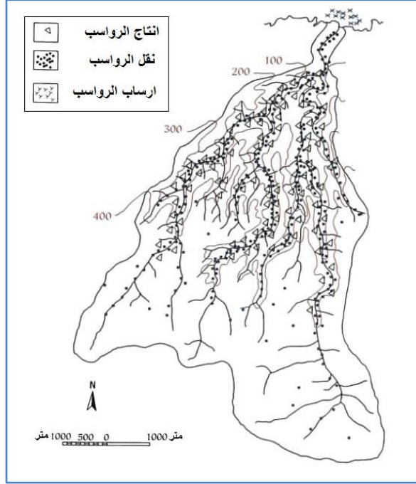
شكل (4) الآليات المقترحة لإنتاج ونقل وترسيب الرواسب في وادي الأثرون بعد عملية ارساب رواسب المصاطب..
