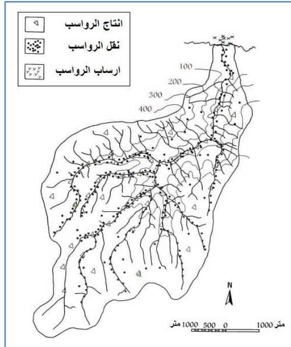
شكل (5) الآليات المقترحة لإنتاج ونقل وارساب الرواسب في وادي مرقص قبل عملية ارساب رواسب المصاطب.
