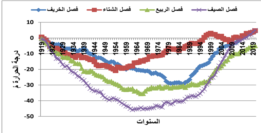
الشكل (11) الفروقات التراكمية لدرجة الحرارة الفصلية الجافة في منطقة طرابلس للفترة 2020-1919م.
