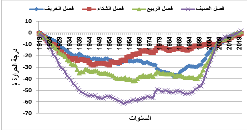
الشكل (9) الفروقات التراكمية لدرجة الحرارة الفصلية العظمى في منطقة طرابلس للفترة 1919-2020م.
