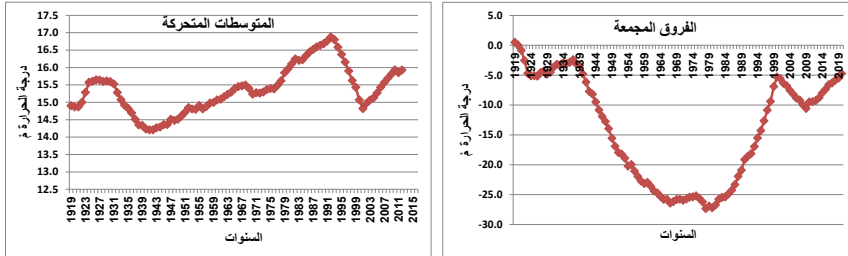
الشكل (4) الفروق التراكمية والمتوسطات المتحركة لدرجة الحرارة السنوية الصغرى في منطقة طرابلس للفترة 1919-2020م.
