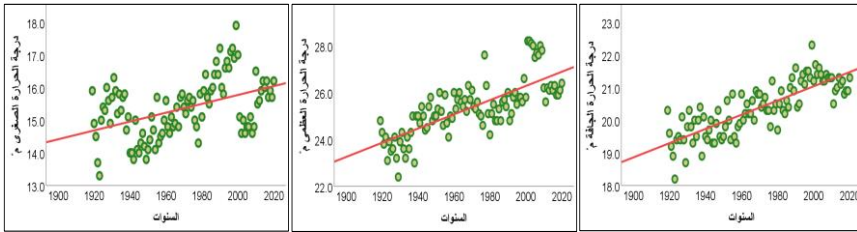
الشكل (5) الانحدار الخطي للمعدل السنوي لدرجة الحرارة الصغرى والعظمى في منطقة طرابلس للفترة 1919 - 2020م.
